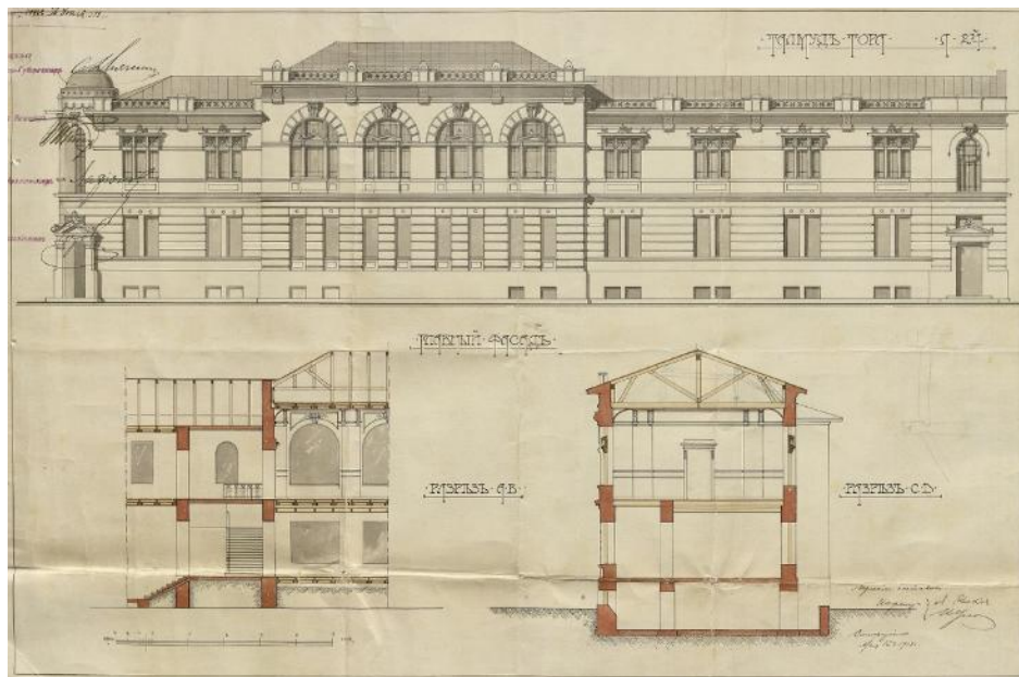
Рис. 7, 8. Проект «общественного еврейского училища Талмуд-Торы в г. Симферополе, угол Лазаретной и Госпитальной». Архитекторы – Я. А. Рыков, В. Ф. Кюблер (?). 12 мая 1913 г. Утвержден на заседании Строительного отделения Таврического губернского правления 2 июля 1913 г. (ГАРК. Ф. 27. Оп. 13. Д. 4785. Л. 4, 5)
