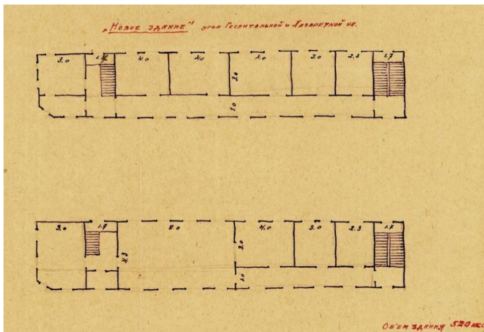
Рис. 15. Планы 1-го и 2-го этажей Талмуд-Торы – «нового здания» Крымского университета им. М. В. Фрунзе. С указанием размеров помещений. Из «Сведений о помещениях, занимаемых Крымским университетом», 1923 г. (ГАРФ. Ф. А-2306. Оп. 70. Д. 9857. Л. 13)
