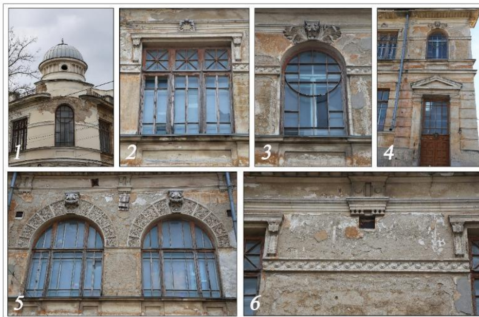
Рис. 13. Конструктивные и декоративные элементы здания Талмуд-Торы: 1. Угловой южный участок с бельведером; 2. Окно главного фасада с прямоугольным сандриком; 3. Оформление оконного проема северной части главного фасада; 4. Входная группа и окно второго этажа северной части главного фасада; 5. Оформление оконных проемов ризалита главного фасада; 6. Декоративная деталь второго этажа главного фасада. Фотоснимки Д. А. Ломакина, 2026 г.
